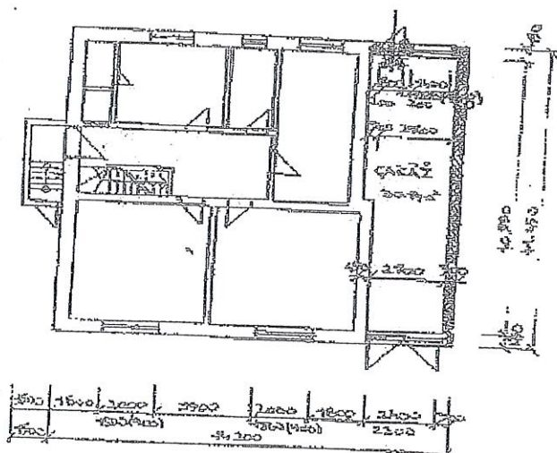
FODORYS PRŮZEMIA M 1:100
